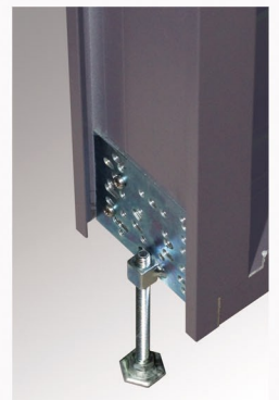
加強板與安裝腳架
